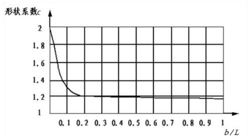
图 4 迎风面形状系数曲线图
