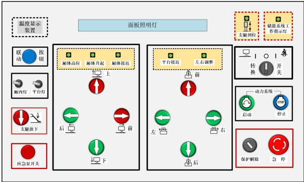
图 2 车厢内部操纵布局示意图
